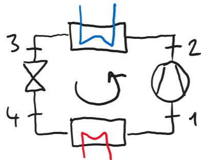
Wärmepumpe / Kältemaschine
