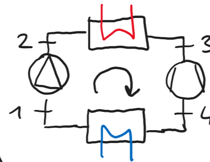
Dampfkräftprozess
