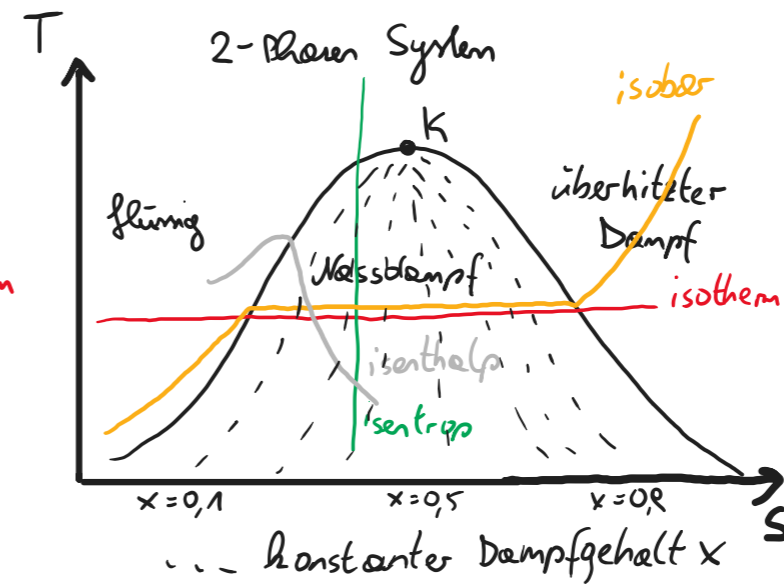
Dampfkräftprozess
